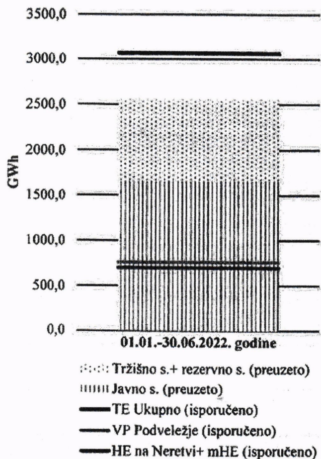
Слика 1. ЈП Електропривреда БиХ д.д. - Сарајево: Остварење производње и потрошње електричне енергије
